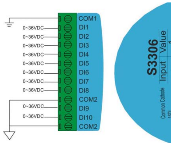
图 1 电压输入
